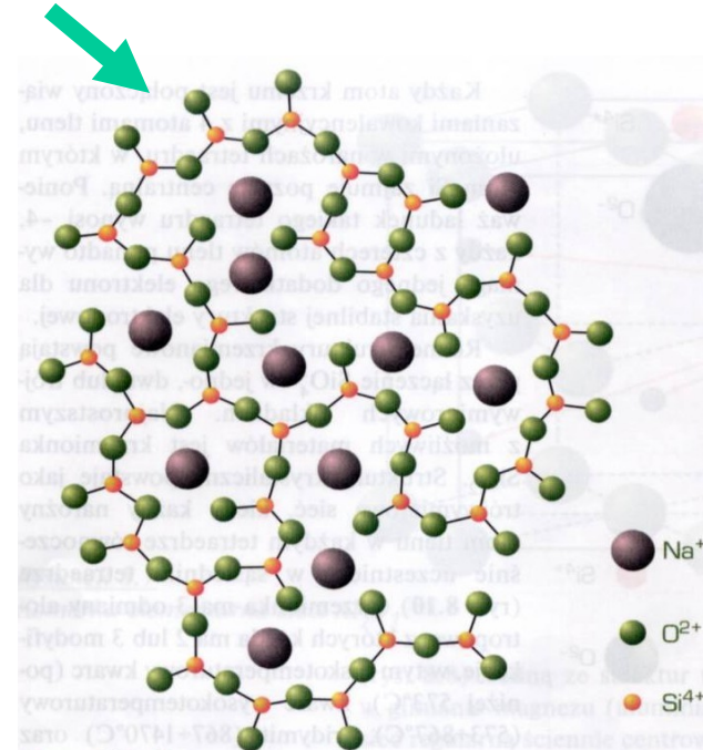
Schemat rozmieszczenia jonów w szkle sodowo-krzemianowym
